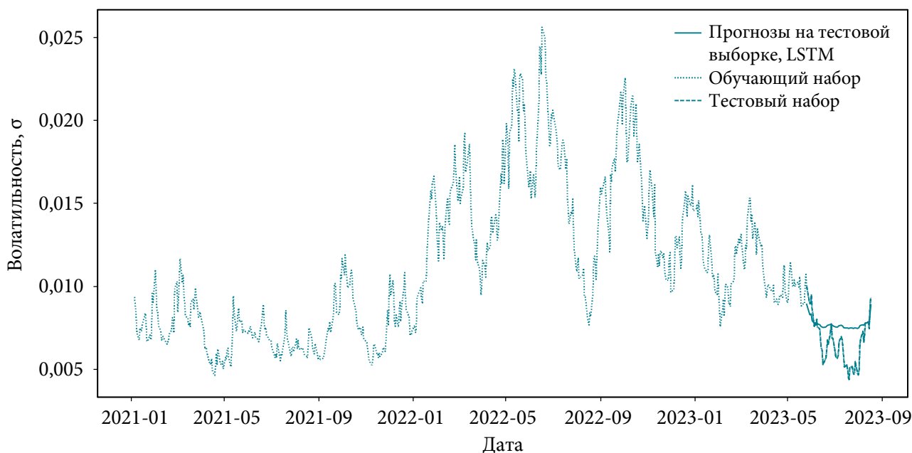
Рис. 3. Прогноз волатильности с помощью LSTM-сети
